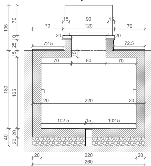
Presjek B-B
