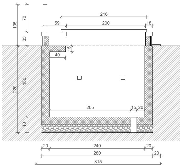
Presjek A-A
