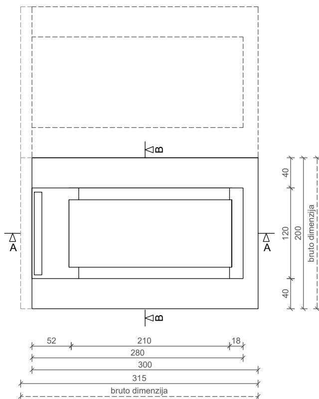
Tlocrt
