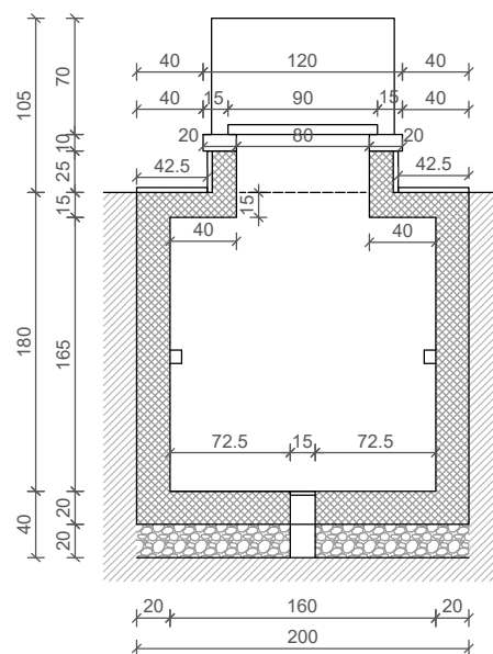
Presjek B-B
